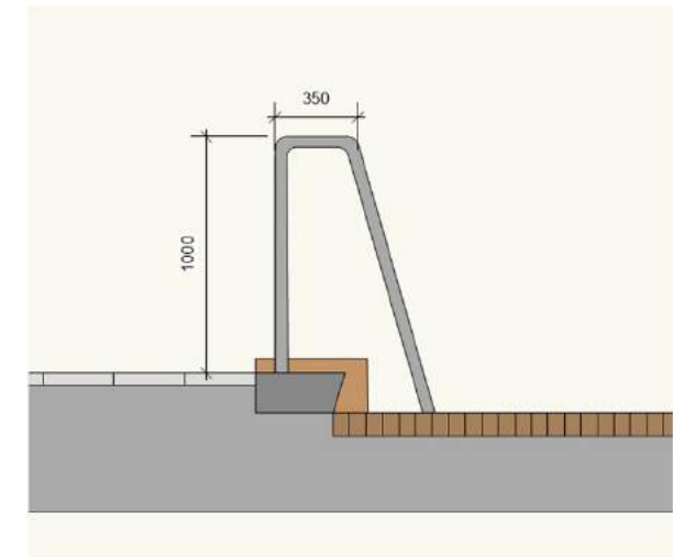
Trapje noordzijde
